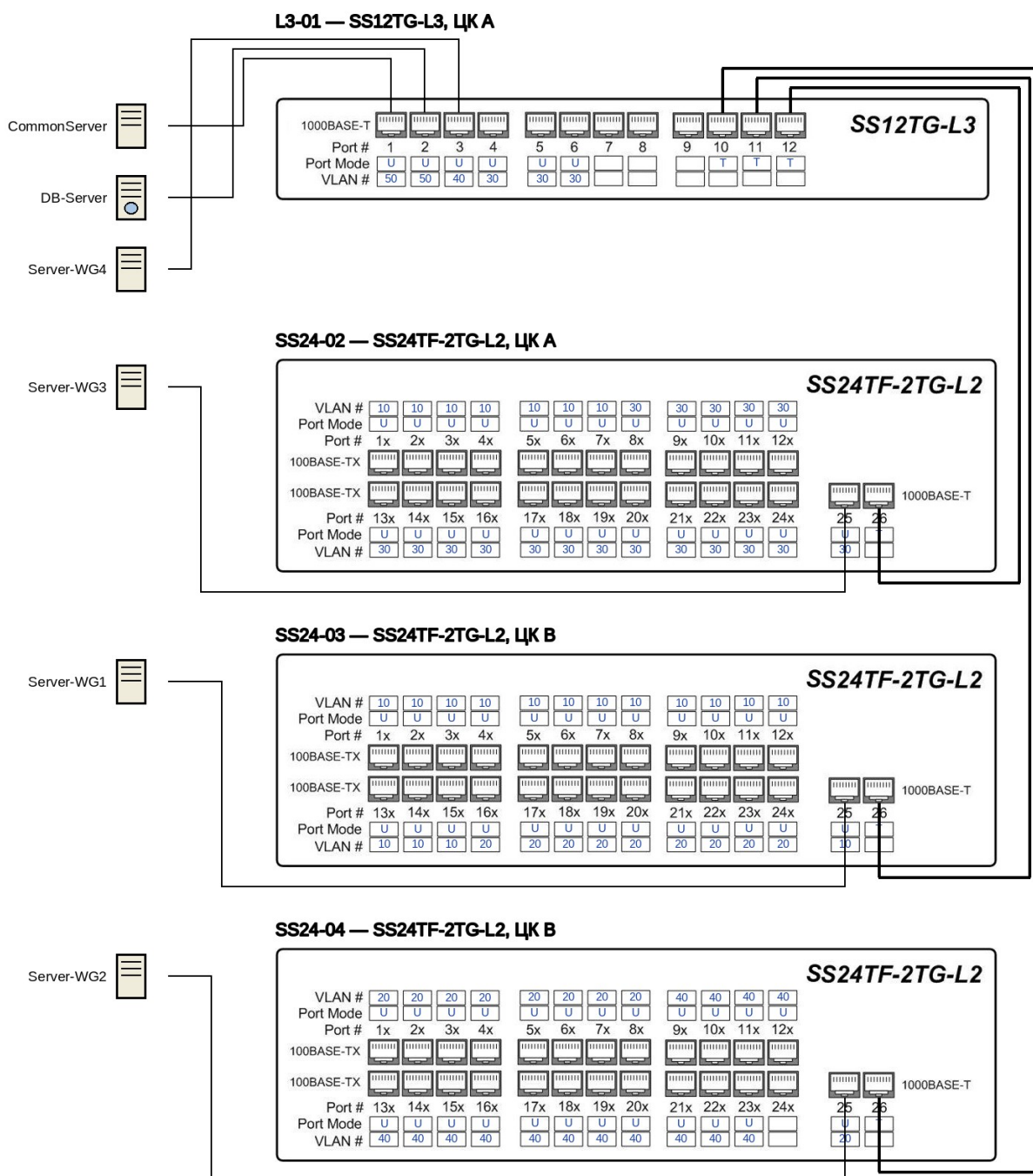
Рисунок 4 – Структура ЛВС с VLAN на интеллектуальных коммутаторах
